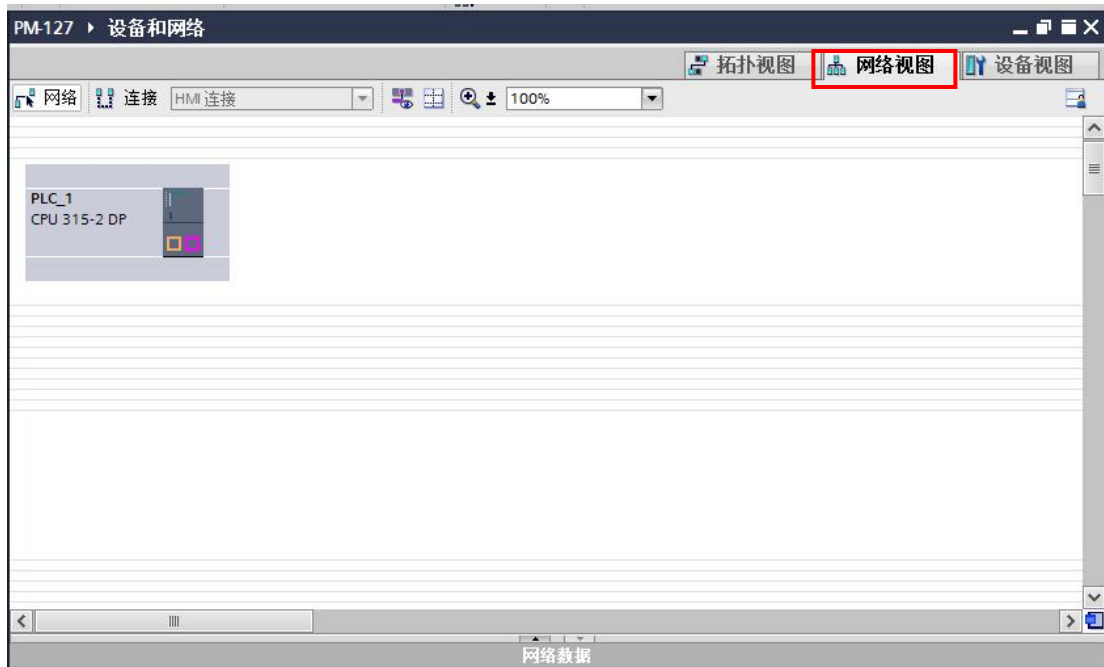
图 15 网络视图
