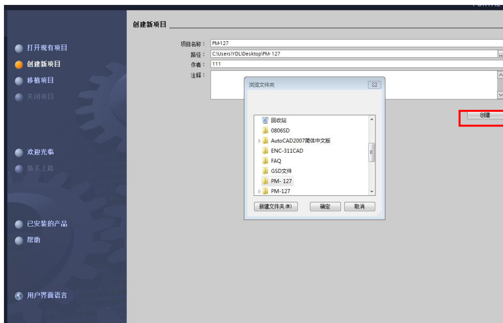
图 2 创建新项目
