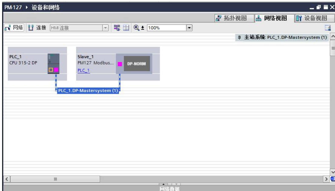
图 19 建立连接
