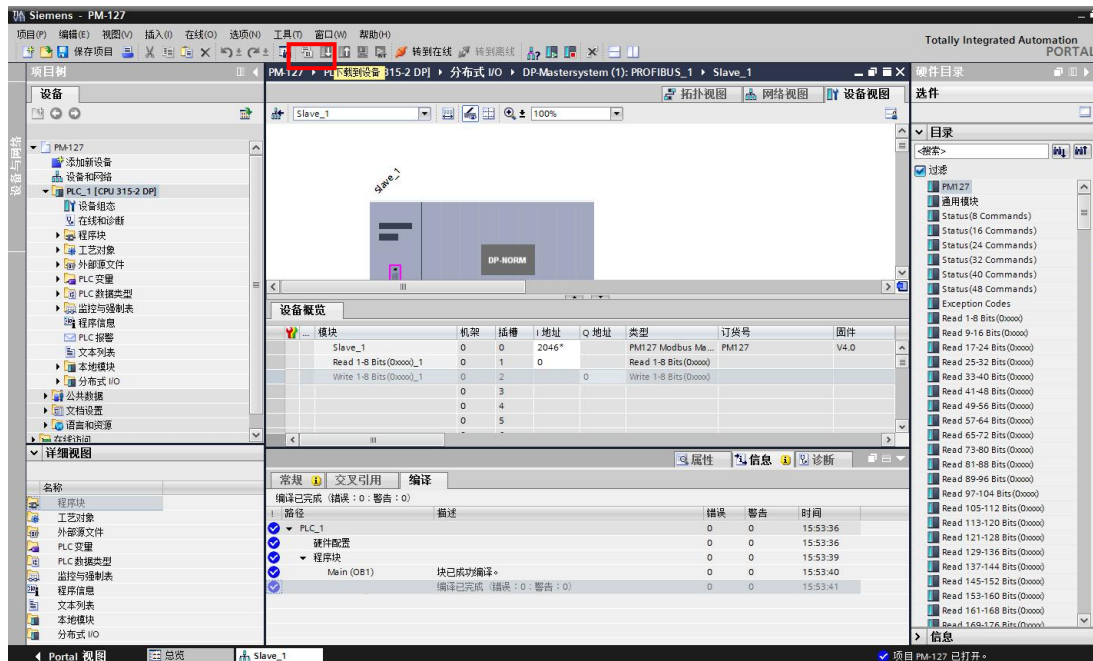
图 24 编译下载
